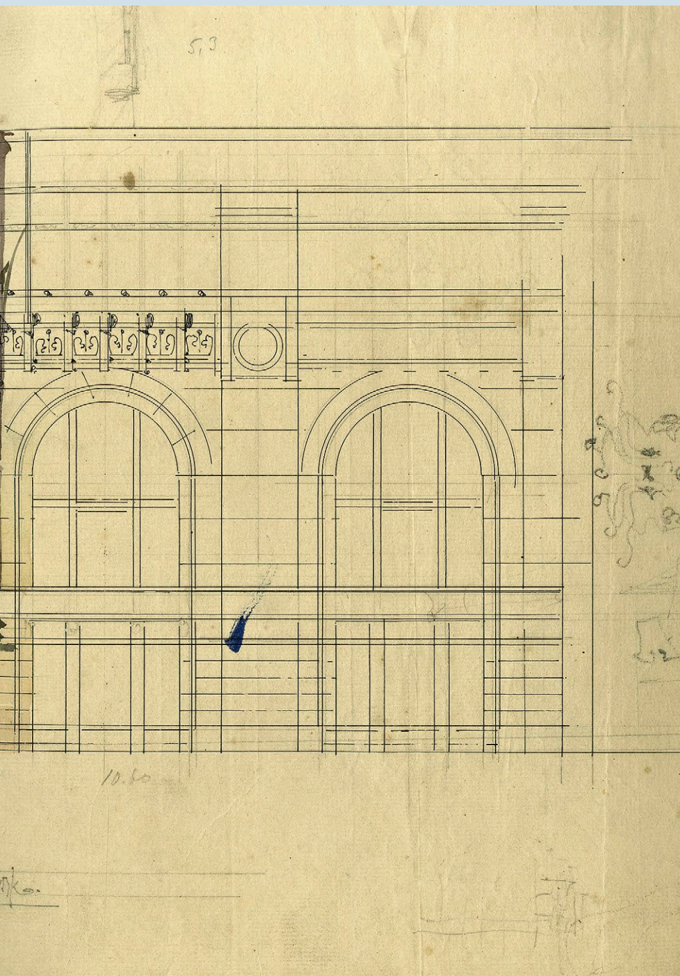
Эскиз с разработкой элементов фасада гостиницы «Метрополь», 1901–1904 годы КККМ, в/ф 6011/43
