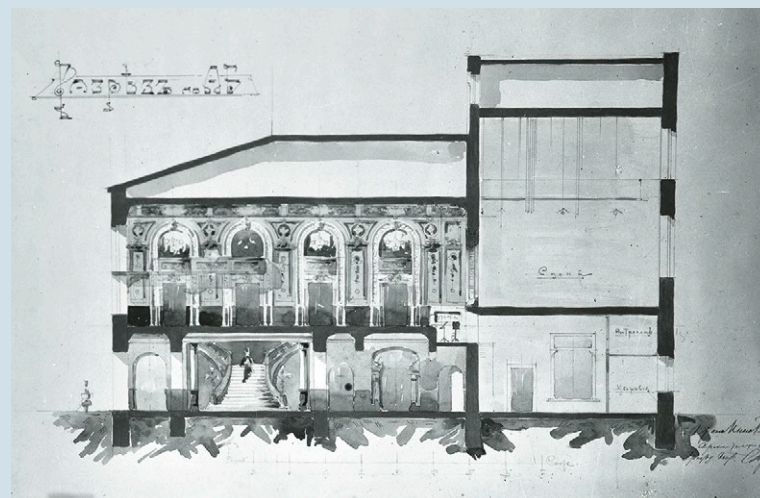
Разрез здания городского театра, 1910-е годы Негатив (пересъемка с проекта) Л. А. Чернышева
