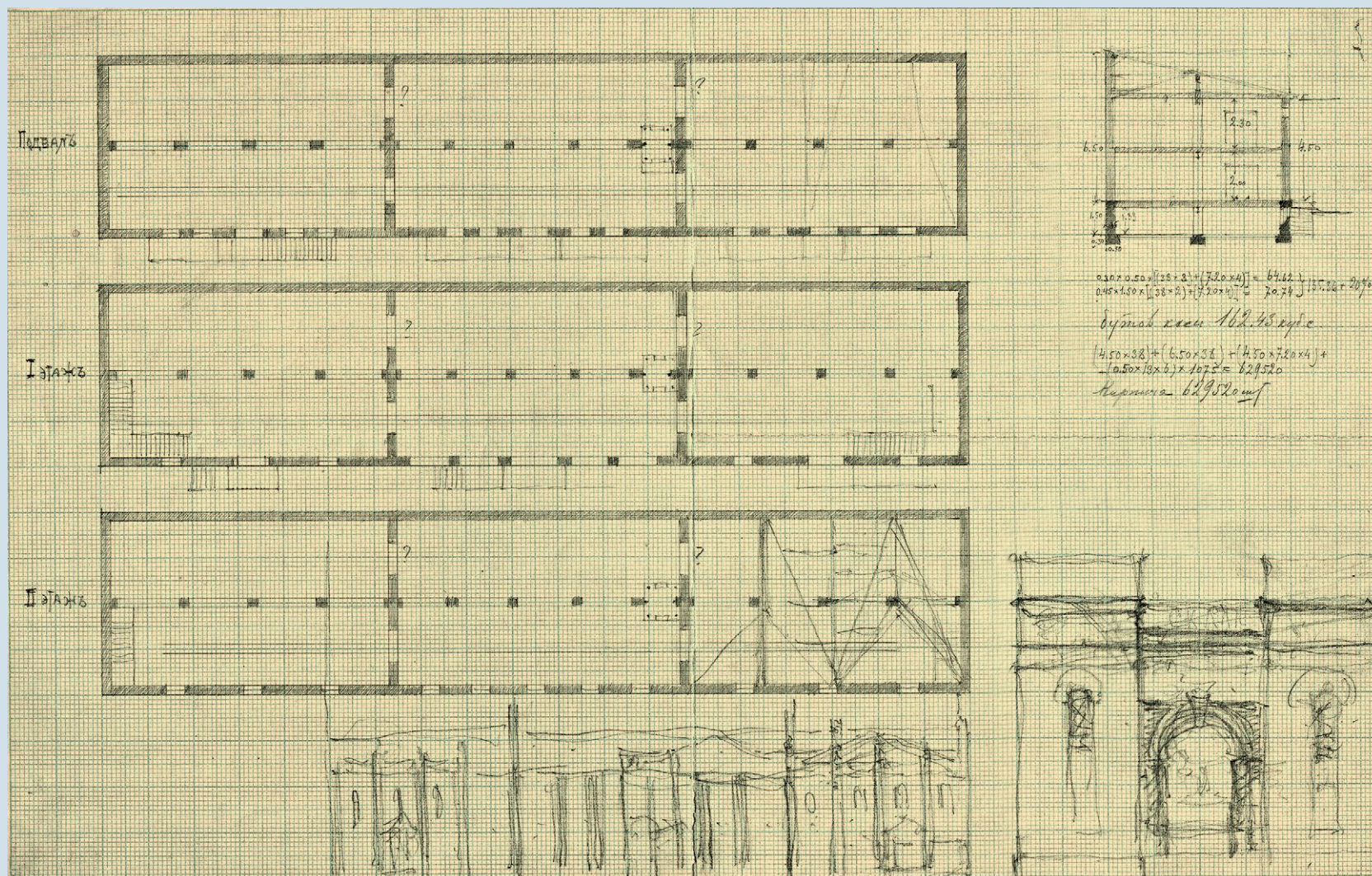
Поэтажный план, боковой разрез и эскиз главного фасада здания складов Енисейского губернского союза кооперативов, 1919–1920 годы ККМ
