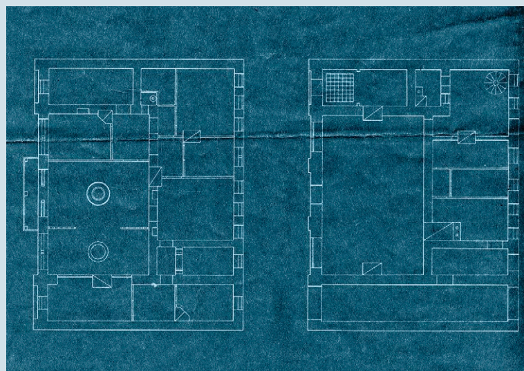
Проект первого и второго этажей дома Бородкина в Енисейске, 1908–1909 годы Копия в технике цианотипия КККМ, в/ф 6011/29
