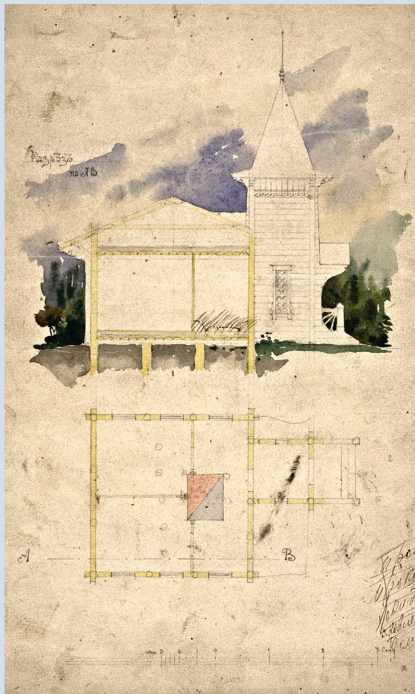
Разрез и план деревянного дома с печным отоплением для омской выставки КККМ, о/ф 10742/4
