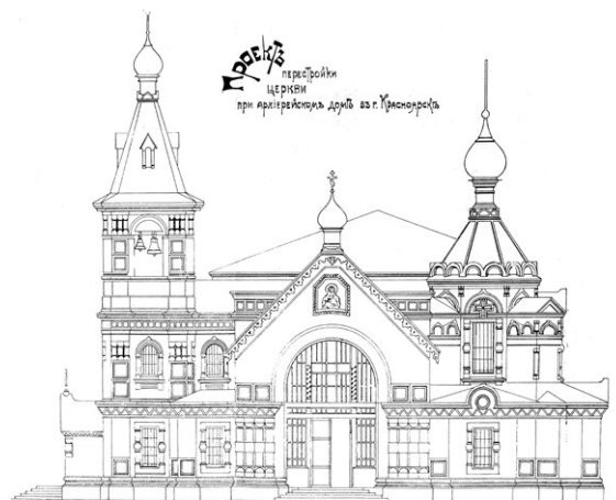
Проект перестройки церкви при Архиерейском доме в Красноярске
