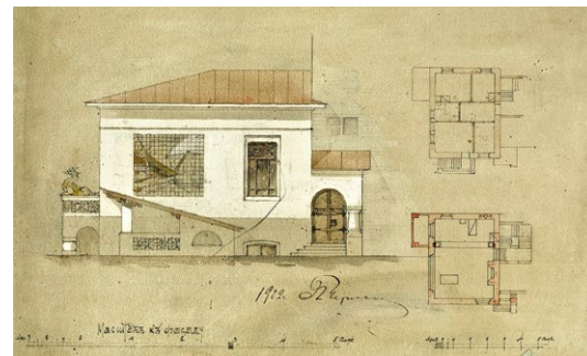
Проект одноэтажного дома с подвальным этажом, 1902 год КККМ, о/ф 8548/11
