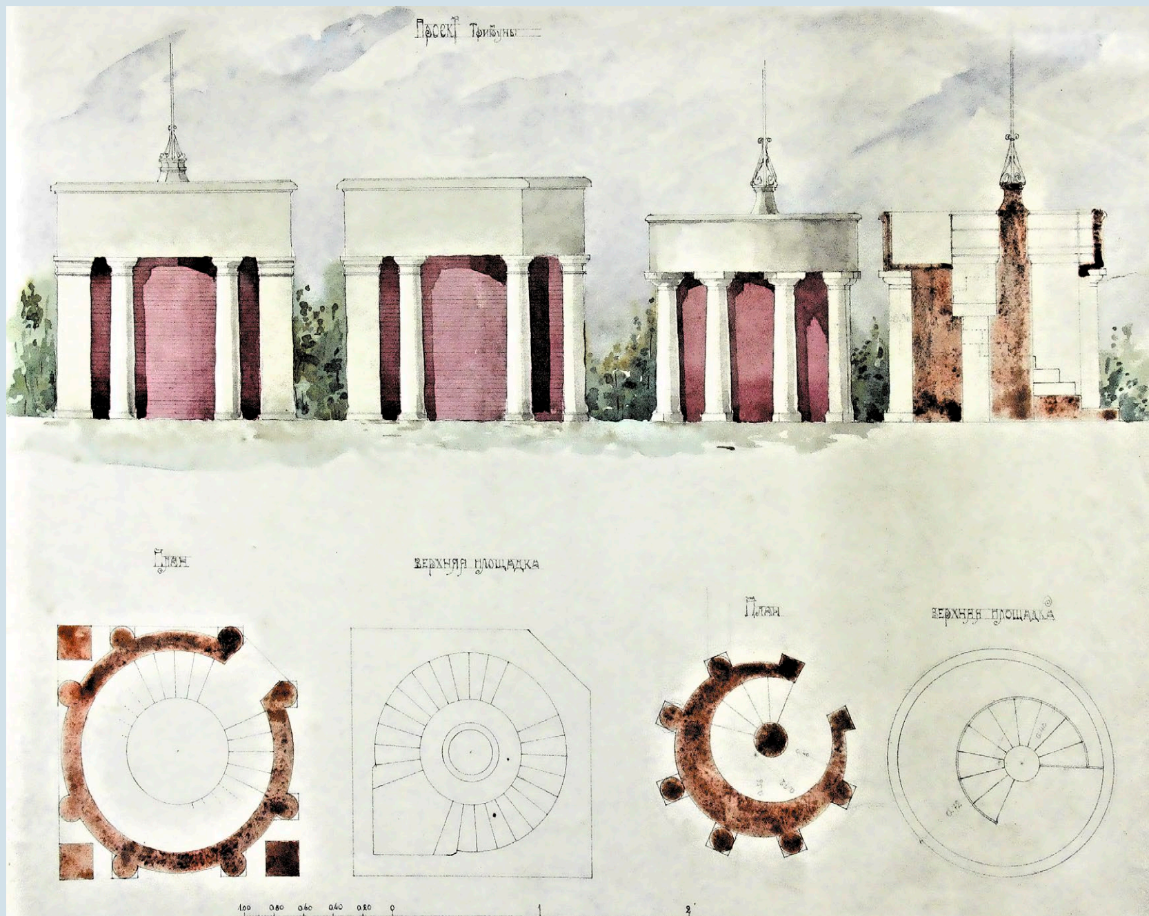
Проект трибун для площади около памятника В. И. Ленину, 1924 год КККМ, о/ф 8891/8
