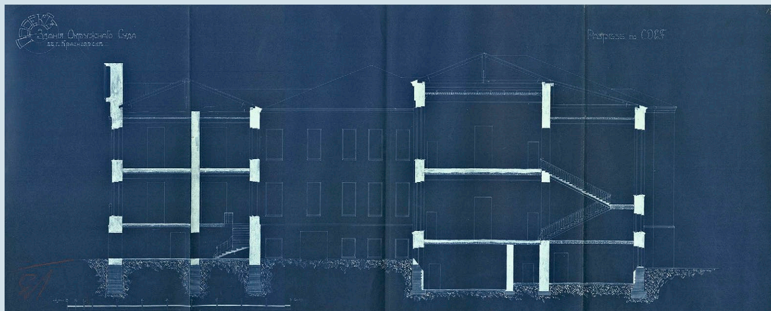
Проект здания Красноярского окружного суда, 1914 год
