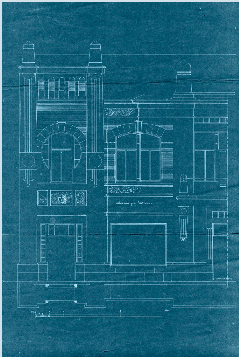
Проект левой части главного фасада дома Бородкина в Енисейске, 1908–1909 годы Копия в технике цианотипия КККМ, в/ф 6011/28
