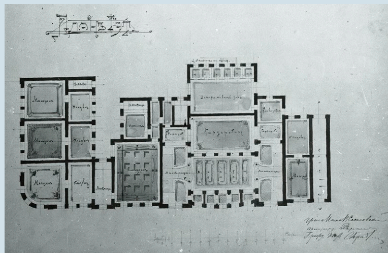
План первого этажа здания городского театра, 1910-е годы Негатив (пересъемка с проекта) Л. А. Чернышева
