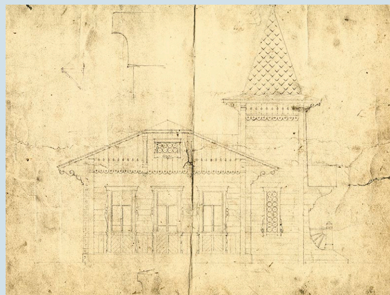
Эскиз бокового фасада деревянного дома с печным отоплением для омской выставки КККМ
