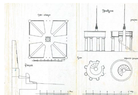
Проект постамента памятника В. И. Ленину, ограды и трибун на площади Революции. 1924 год КККМ, в/ф 12172/13
