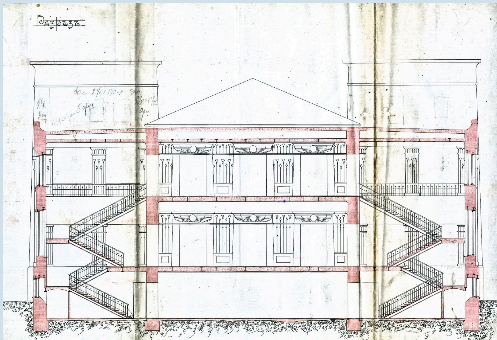
Проект городского музея, 1912 год КККМ
