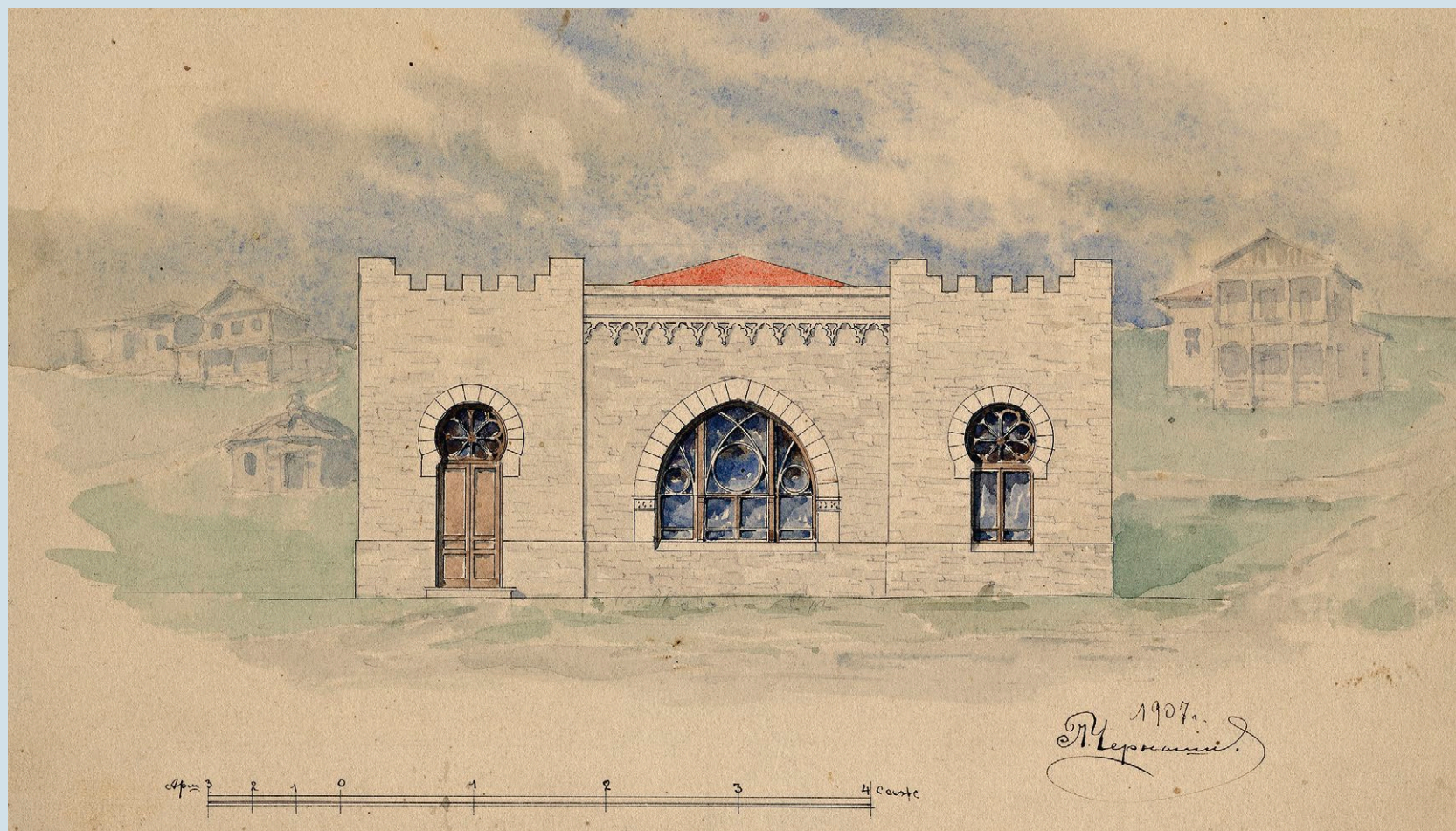
Л. А. Чернышев. Эскизный проект здания приемного покоя для курорта на озере Шира, 1907 год КККМ, о/ф 8777/16
