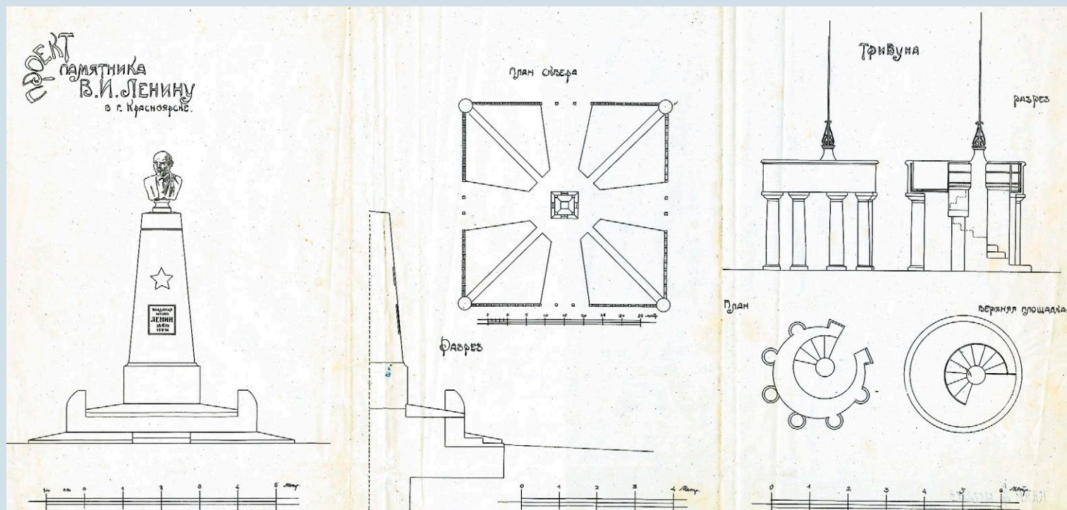
Проект постамента памятника В. И. Ленину и трибун на площади около памятника в Красноярске, 1924 год КККМ, в/ф 12172/13
