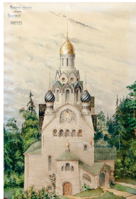
Проект церкви на 300 человек, северный фасад, 1905 год КККМ, ПГС 764
