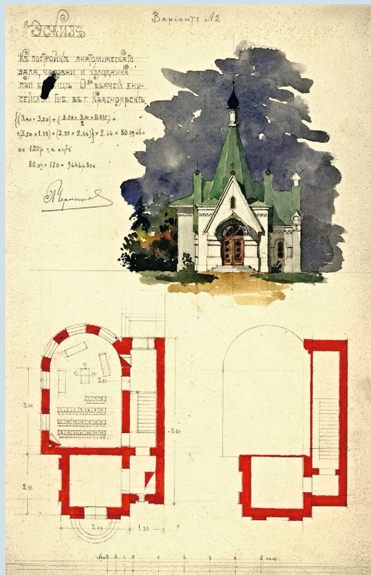
Эскиз к постройке анатомического зала, часовни и холодильника при больнице Общества врачей Енисейской губернии в Красноярске, 1910-е годы
