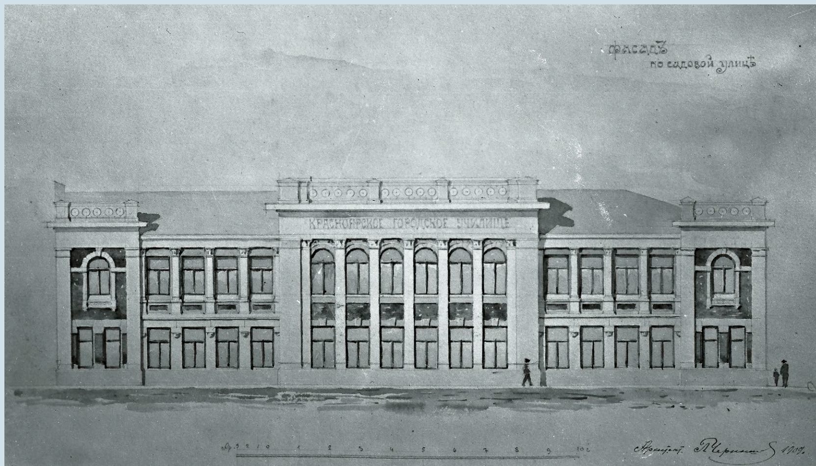
Проект четырехклассного городского училища, фасад по Садовой улице, 1909 год Негатив (пересъемка с проекта) Л. А. Чернышева КККМ
