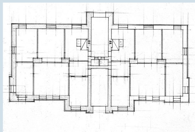
Проект главного фасада и планы первого и второго этажей неустановленного здания, 1910-е годы КККМ
