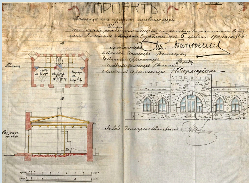
Л. А. Чернышев. Утвержденный проект больницы при курорте озера Шира, 1910 год
