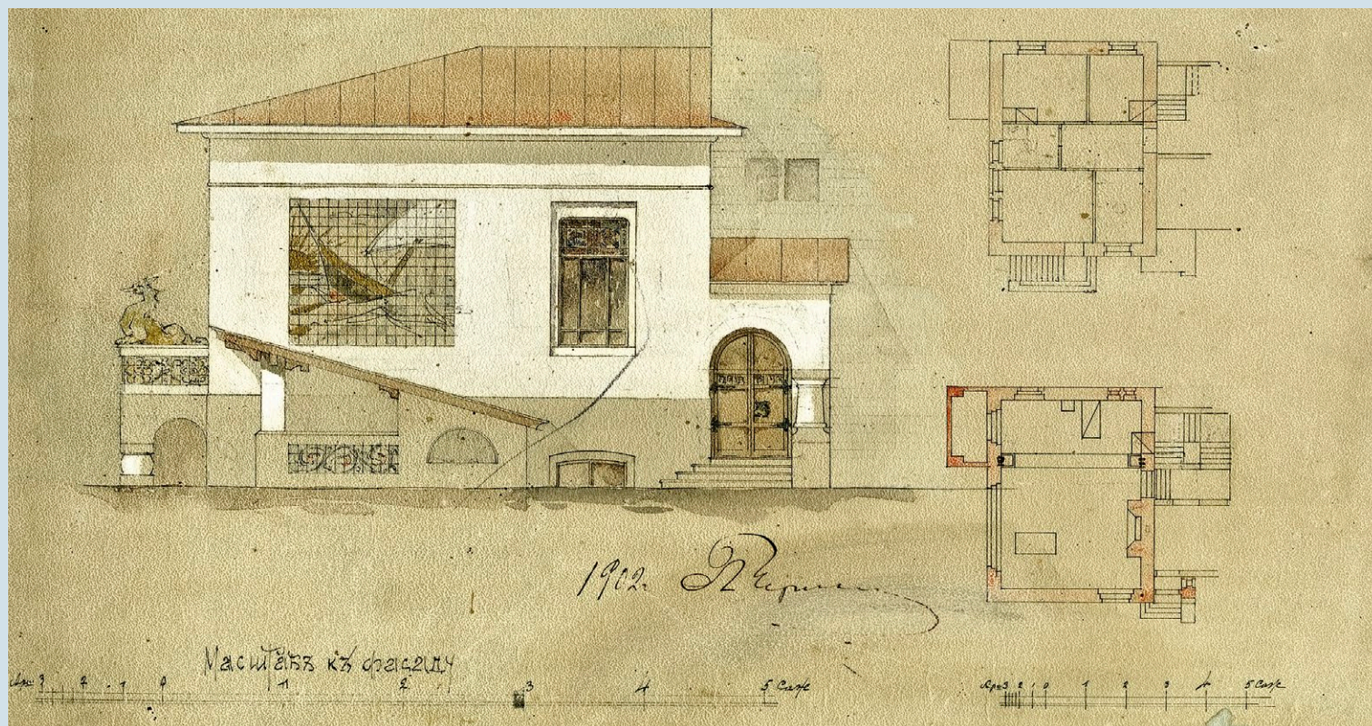
Проект небольшого особняка с подвальным этажом, 1902 год КККМ, о/ф 8548/11
