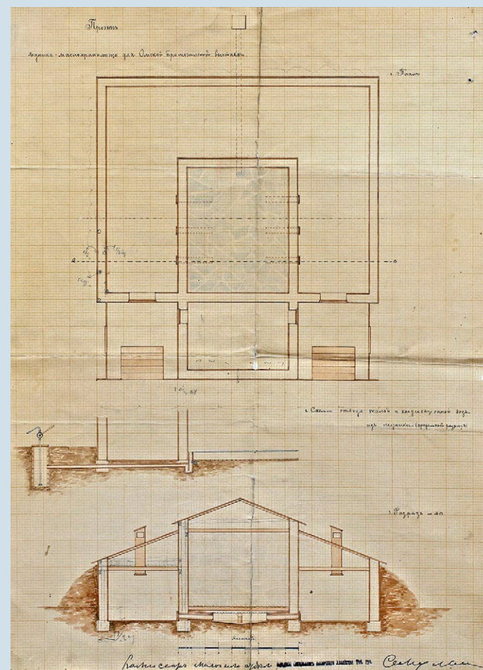
Проект ледника-маслохранилища для омской выставки, 1911 год КККМ, о/ф 8777/9
