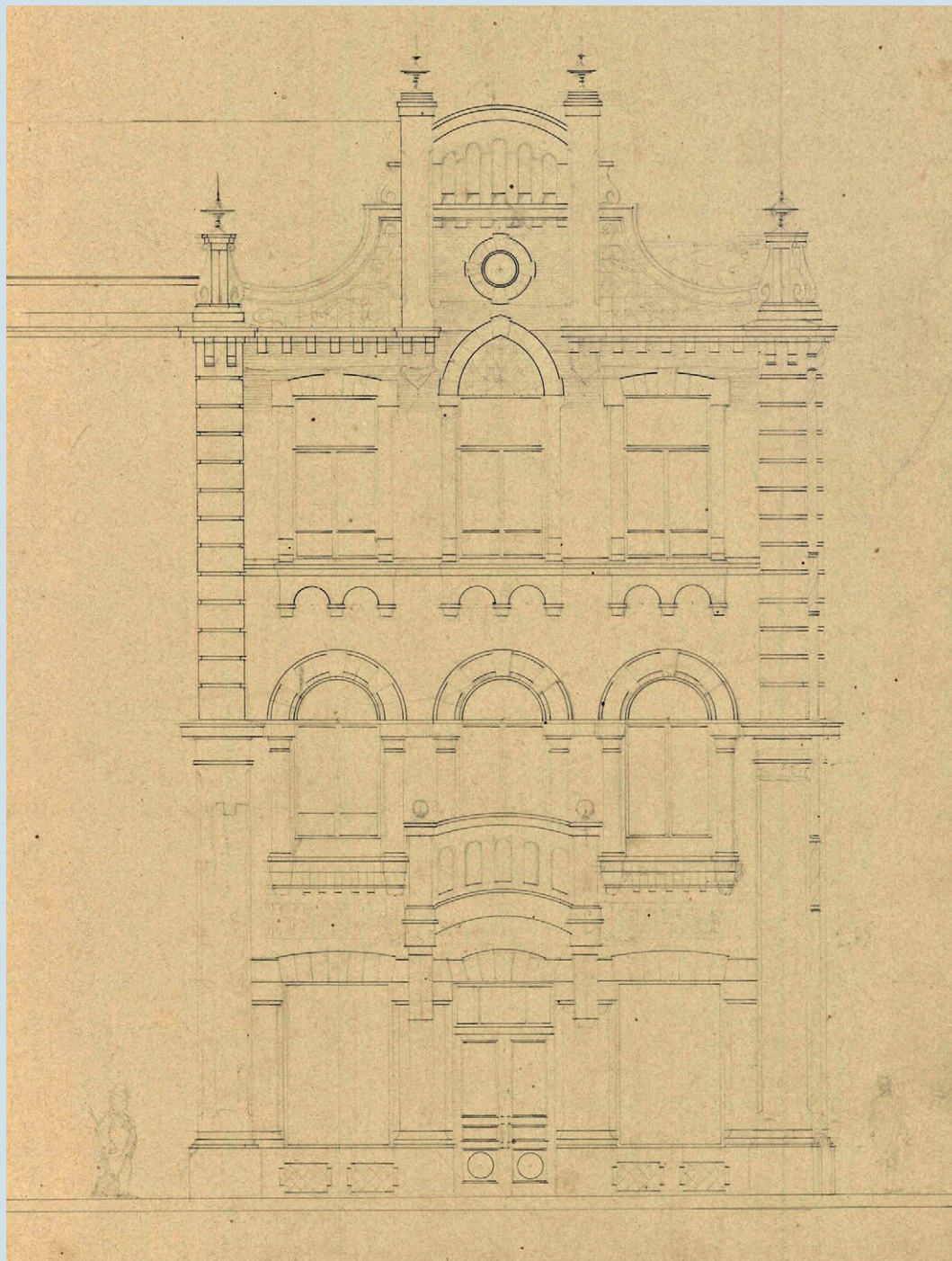
Проект дома купеческого общества, эскиз части фасада с ризалитом, 1908 год ГАКК. Ф. 796. Оп. 1. Д. 4582
