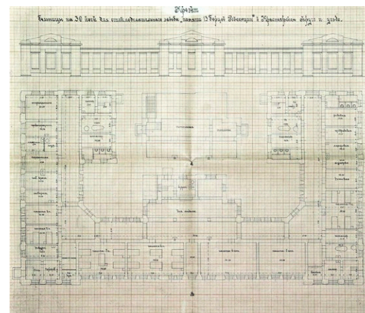
Проект больницы на 30 коек для стекольного завода в поселке Памяти 13 Борцов Революции, 1927 год КККМ, в/ф 6011/24
