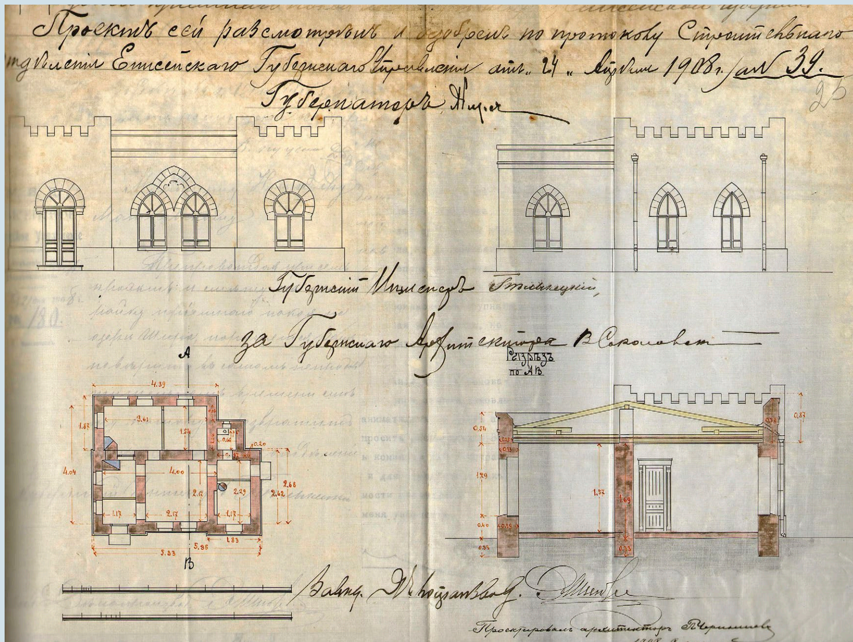
Л. А. Чернышев. Утвержденный проект здания приемного покоя для курорта озера Шира, 1908 год
