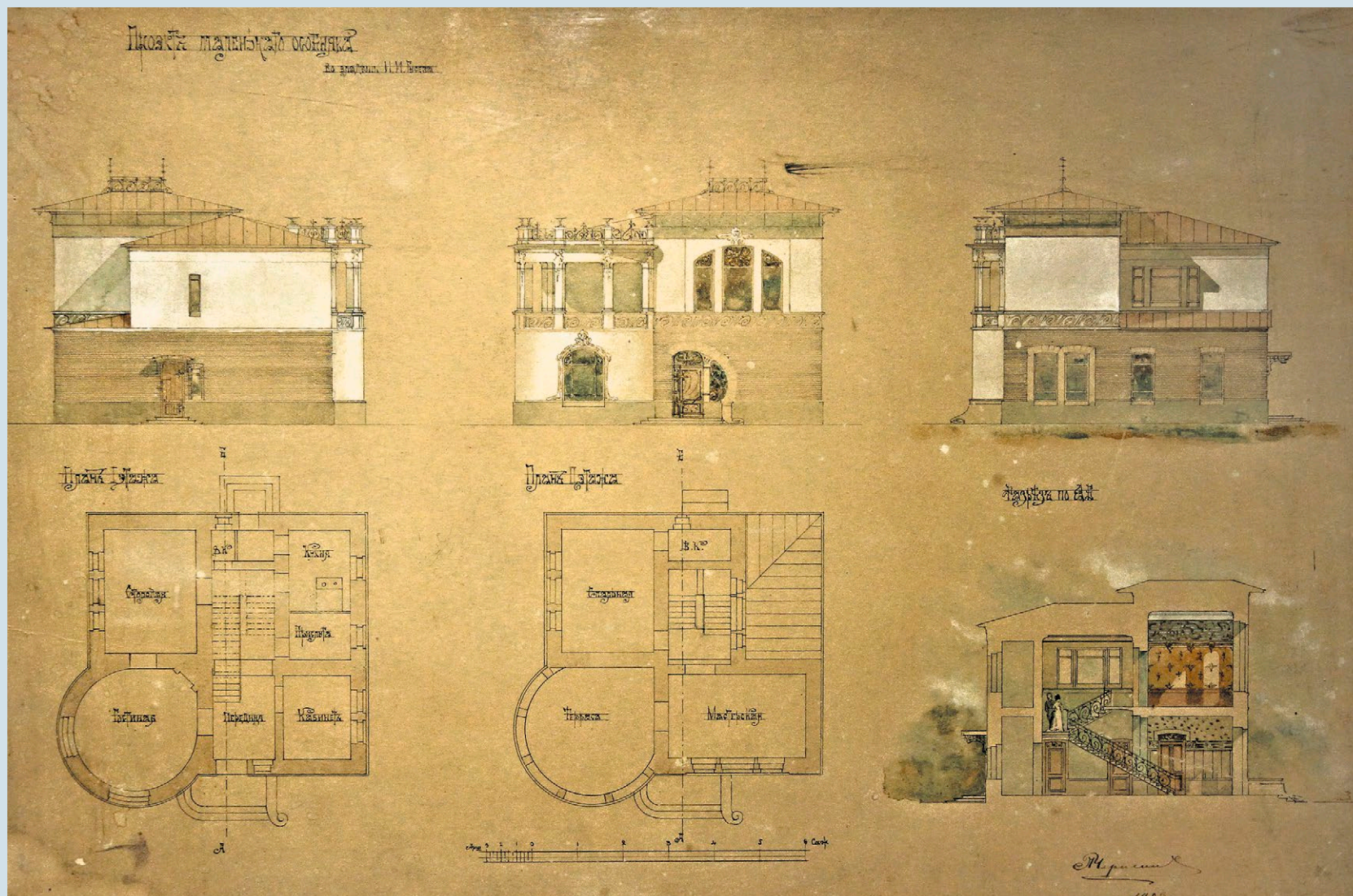
Проект маленького особняка во владении И. И. Гусева, 1903 год ККМ, о/ф 10100/135
