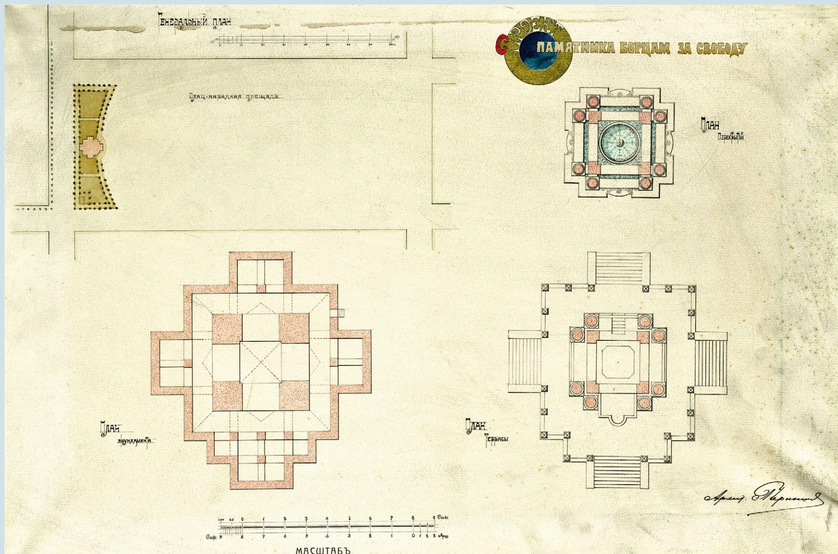
Генеральный план памятника борцам за свободу, 1920-е годы КККМ, о/ф 8548/6
