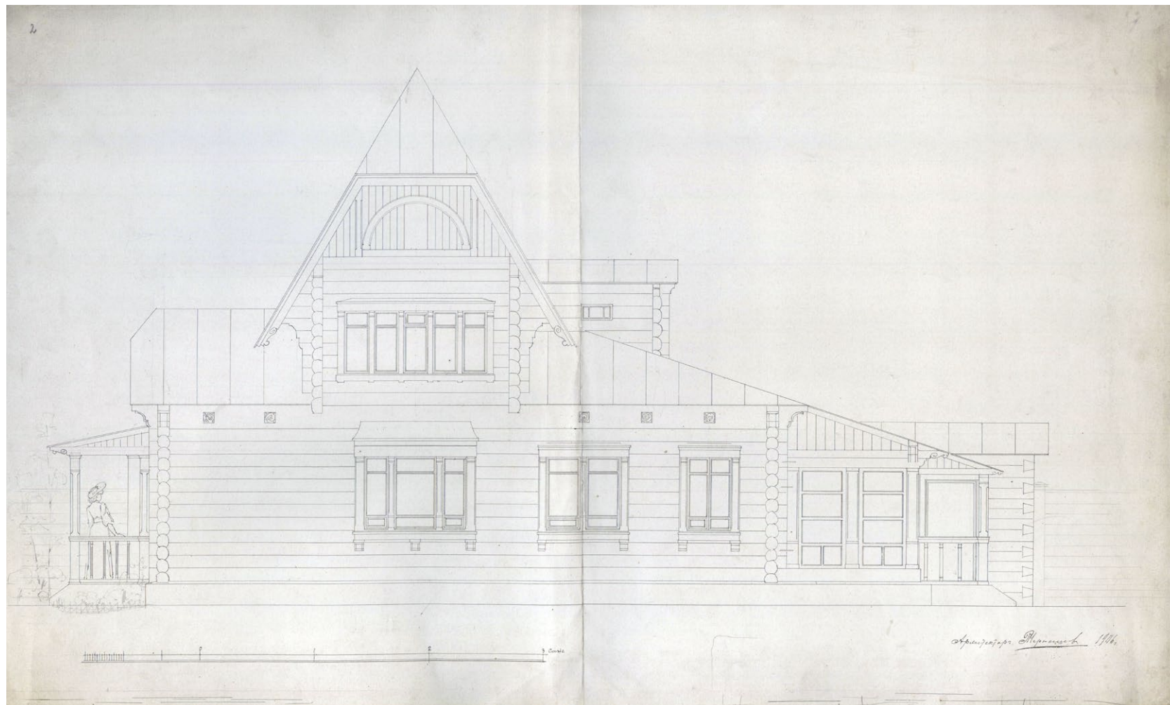
Эскиз западного фасада флигеля. 1906 г. Карандаш. Л. А. Чернышев. ГАКК. Ф. 796. Оп. 1. Д. 4580.
