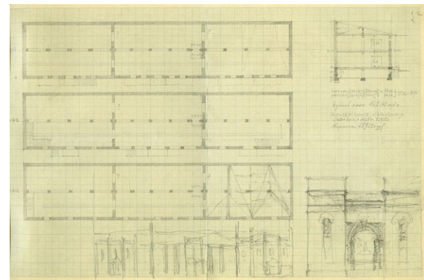
Набросок главного фасада, боковой разрез и поэтажные планы к проекту складов Енисейского губернского союза кооперативов. [1920–1921 гг.]. Карандаш. Л. А. Чернышев. КККМ.
