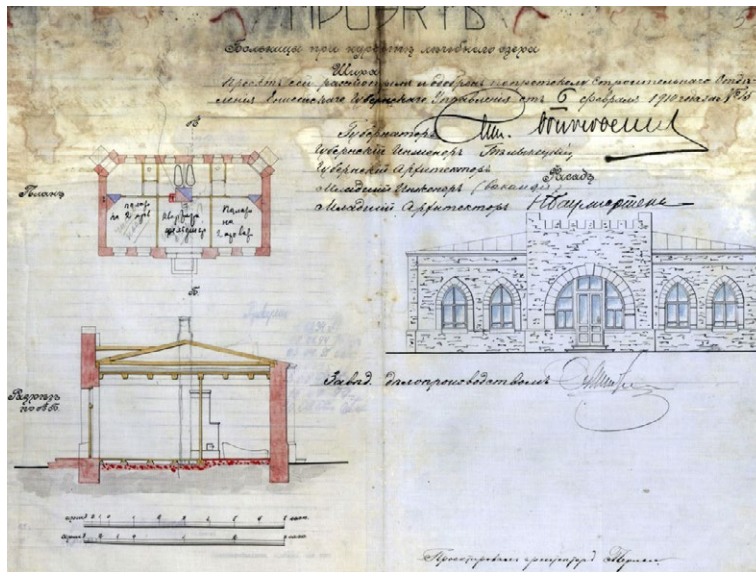
Проект больницы при курорте лечебного озера Шира. 1910 г. Л. А. Чернышев. ГАКК. Ф. 595. Оп. 59. Д. 541. Л. 5.
